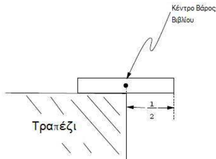
Σχήμα 1: Ένα βιβλίο μπορεί να είναι το πολύ κατά το ήμισυ εκτός τραπέζιου.
