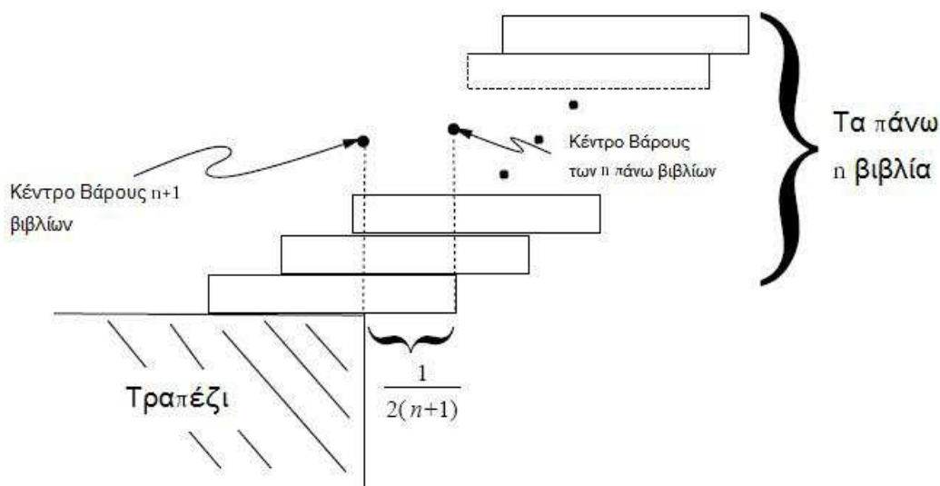
Σχήμα 2: Επιπρόσθετη προέκταση για n + 1 βιβλία.
